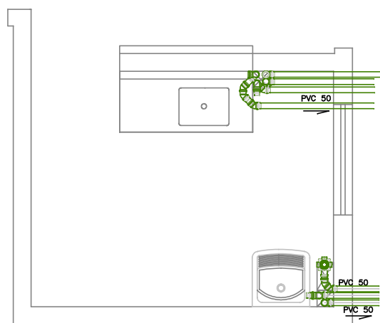
COZINHA — PAVTO. TÉRREO
