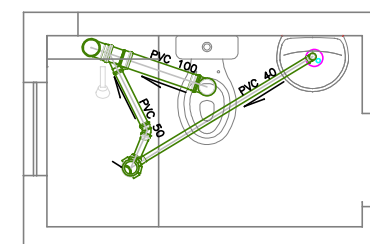
BANHO — PAVTO. TIPO
