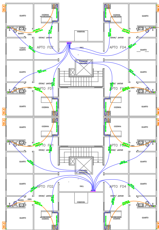
PLANTA PAVIMENTO TIPO BLOCOS 01 A 14
