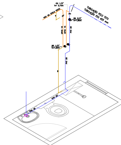
BANHO – ÚLTIMO PAVIMENTO
