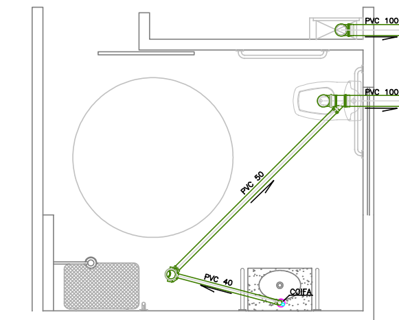
BANHO PNE – PAVTO. TÉRREO
