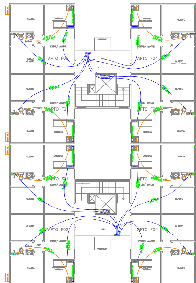
PLANTA ÚLTIMO PAVIMENTO BLOCOS 01 A 14
