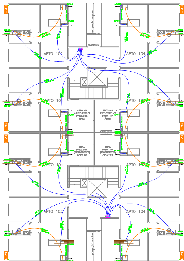
PLANTA PAVIMENTO TÉRREO BLOCOS 01 A 14
