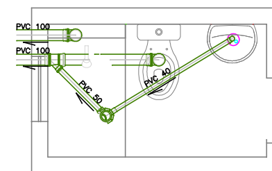
BANHO — PAVTO. TÉRREO
