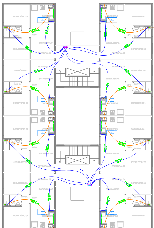
PLANTA PAVIMENTO TIPO BLOCOS 01 A 14
