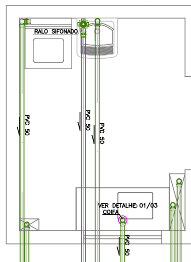
COZINHA — PAVTO. TÉRREO
