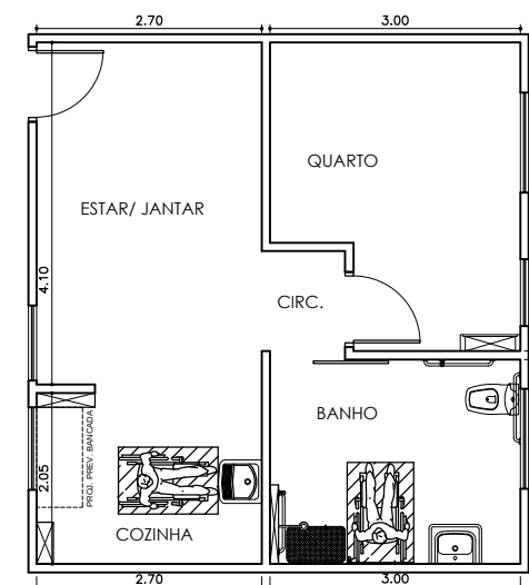
DETALHE DO LAYOUT DOS APARTAMENTOS COM POSSIBILIDADE DE ADAPTAÇÃO BLOCO 08: APTOS 101, 102 E 104.
